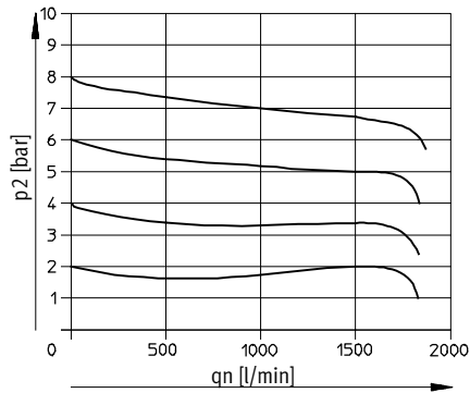
LFR/LFRS-1/4-D-MINI
