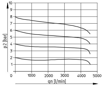
LFR/LFRS-1/2-D-MIDI
